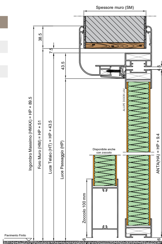
SEZIONE VERTICALE
