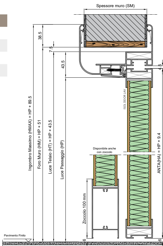
SEZIONE VERTICALE
