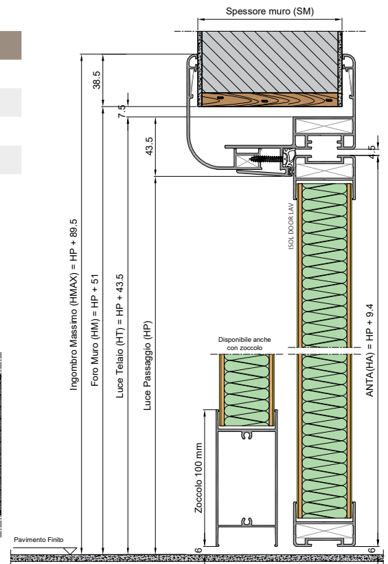
SEZIONE VERTICALE
