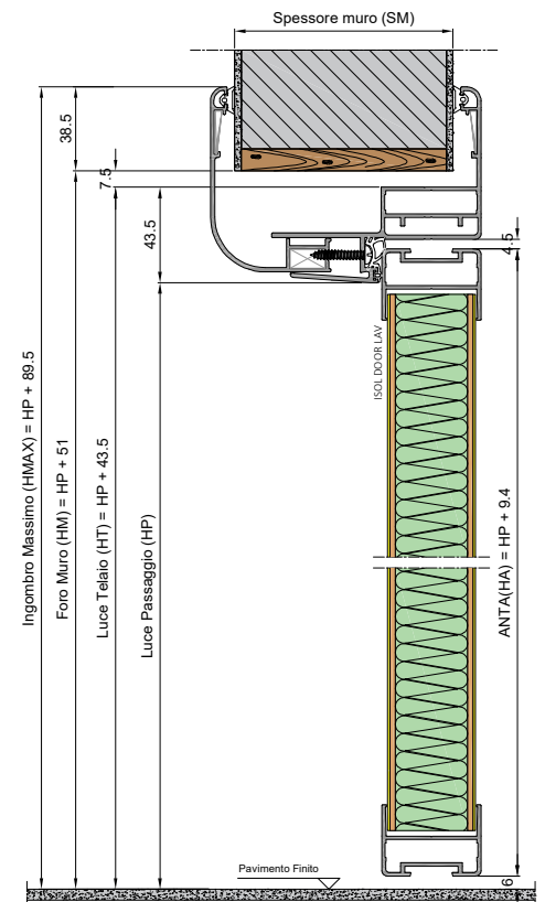
SEZIONE VERTICALE
